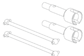
500405937 Antriebswellen-Set (2) Expl. 016 hinten / Dog bone rear (2)
