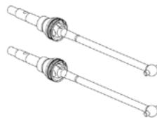
500405936 Antriebswellen vorne (2) Expl. 019 Front drive shafts (2)
